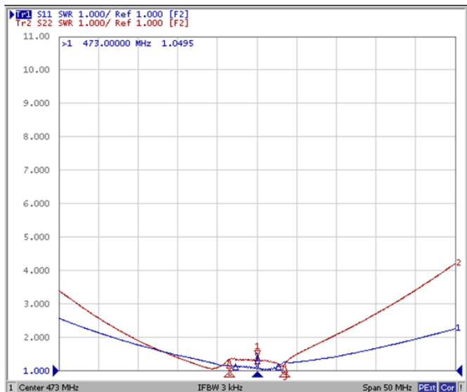
VSWR
