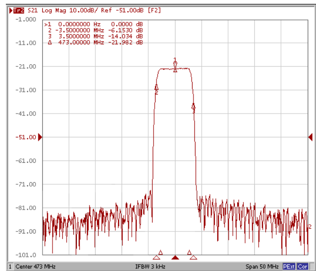
Attenuation (Fo±3.5MHz)
